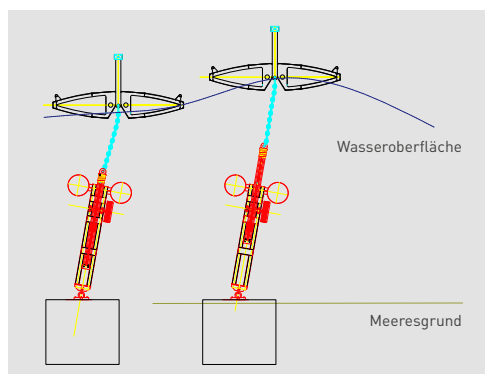
Wirkungsprinzip Energieboje
